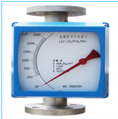
方型指示器
